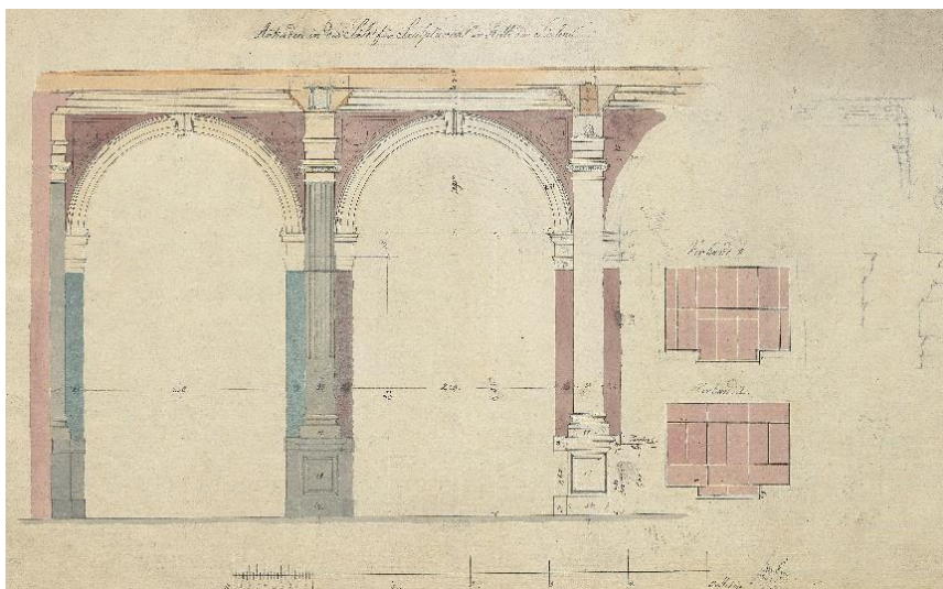
Julius Robert Engers Entwurf der Arkaden in den Sälen des 1. Obergeschosses, Abbildung: Landesarchiv Thüringen – Staatsarchiv Altenburg
